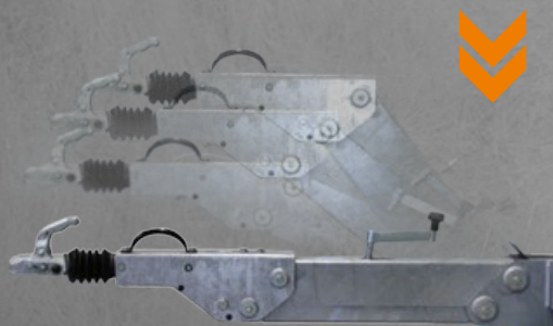
KURBELHÖHENVERSTELLUNG
