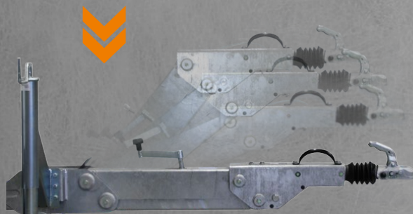
KURBELHÖHENVERSTELLUNG
